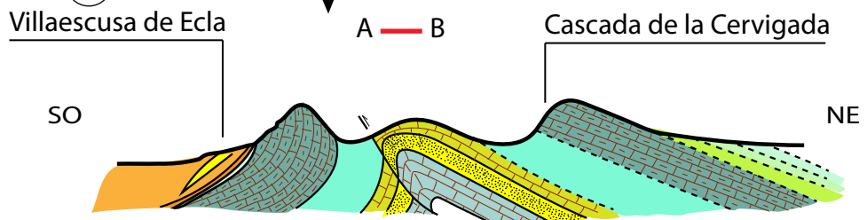
① : Secuencia de imágenes aéreas de la zona del anticlinal de Villaescusa de Ecla donde se ha ido superponiendo la cartografía geológica. ② : Corte geológico A-B
